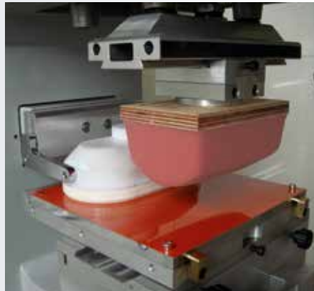
Rakeltopf Kreuztisch
